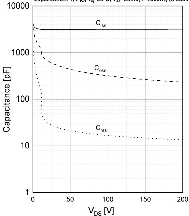
电容
