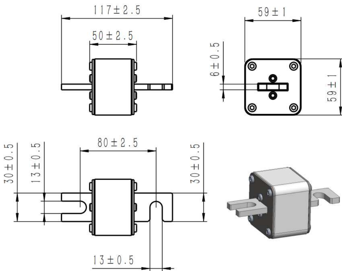
Din: xxxUN-59E 勾叉螺栓横向安装 without fuse indicator
