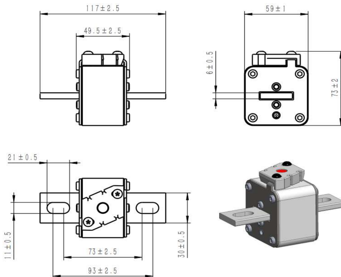
Bolted: xxxB-59E 长条螺栓横向安装
