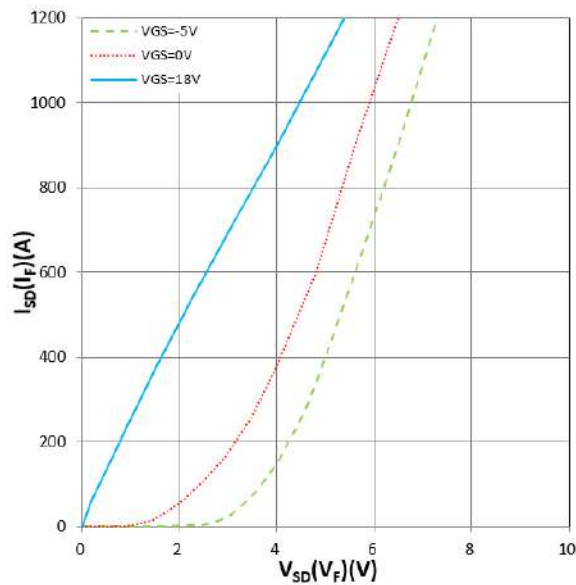
Figure 8. I_{SD}(I_F) vs V_{SD}(V_F) T_j = 175^\circ\text{C} , V_{GS} parameter
