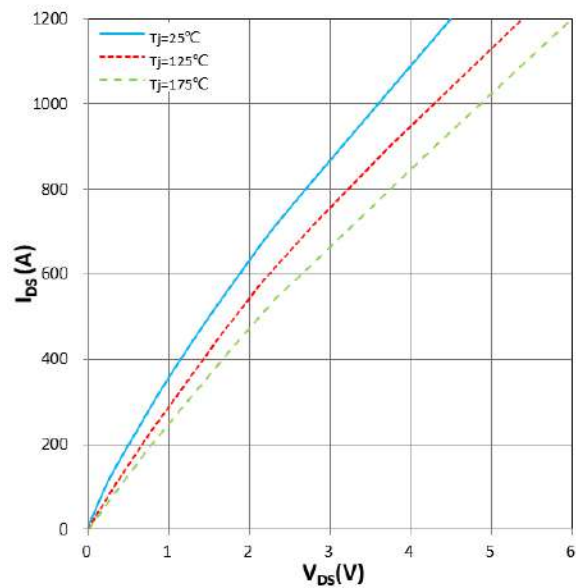
Figure 6. I_{DS} vs V_{DS} V_{GS} = 18\text{V} , T_j parameter
