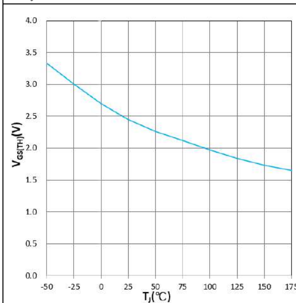
Figure 15. V_{GS(TH)} vs T_J V_{DS} = V_{GS} , I_{DS} = 20\text{mA}
