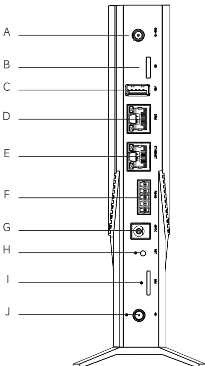
4G Module ( Model: HC-DMU-4G)
