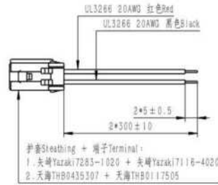
线圈连接器(选配) Coil Connector(Optional)
