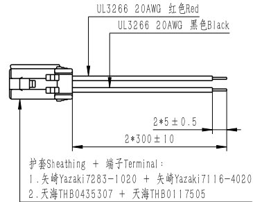
线圈连接器(选配) Coil Connector(Optional)
